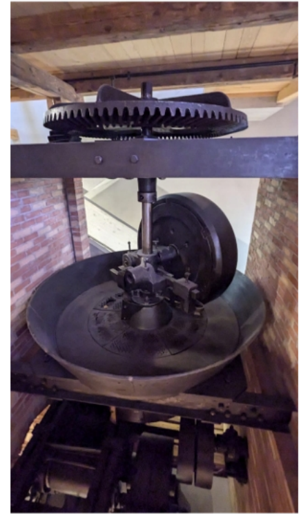
▼▲ Ziegelmaschine im Kunstmuseum/Kunsthalle Appenzell. oben: der Kollergang links: das darunter liegende Walzwerk
