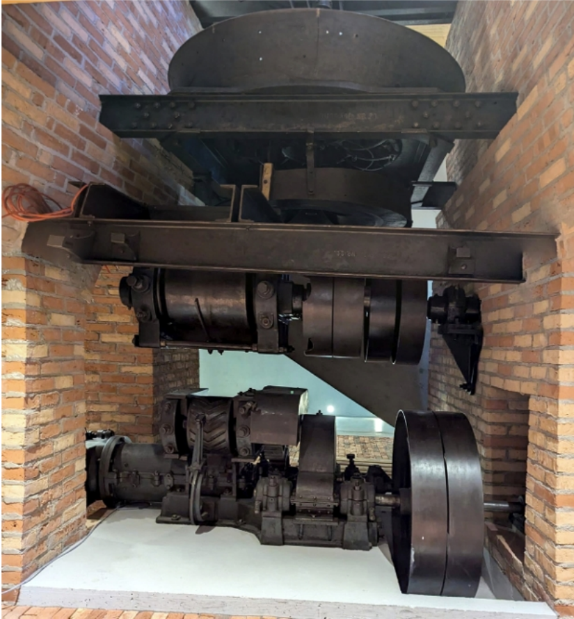
▼▲ Ziegelmaschine im Kunstmuseum/Kunsthalle Appenzell. oben: der Kollergang links: das darunter liegende Walzwerk
